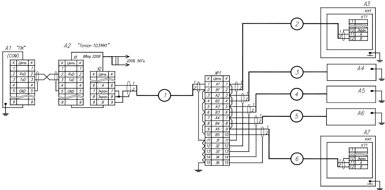
Рис. 1.2. Линия связи ТРК серий "Топаз" по интерфейсу RS-485 последовательного типа.
