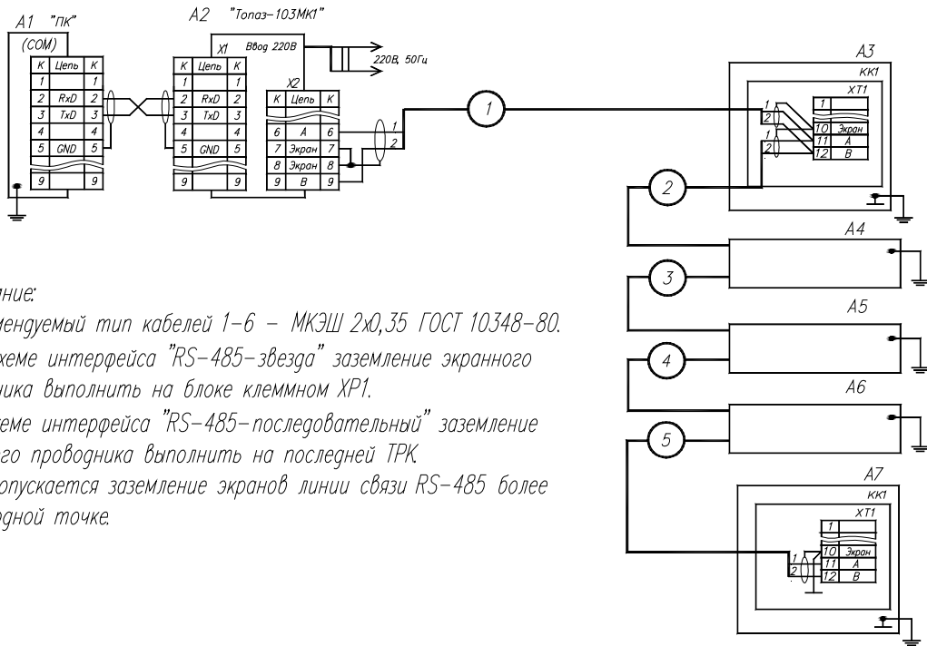
Рис. 1.2. Линия связи ТРК серий "Топаз" по интерфейсу RS-485 последовательного типа.
