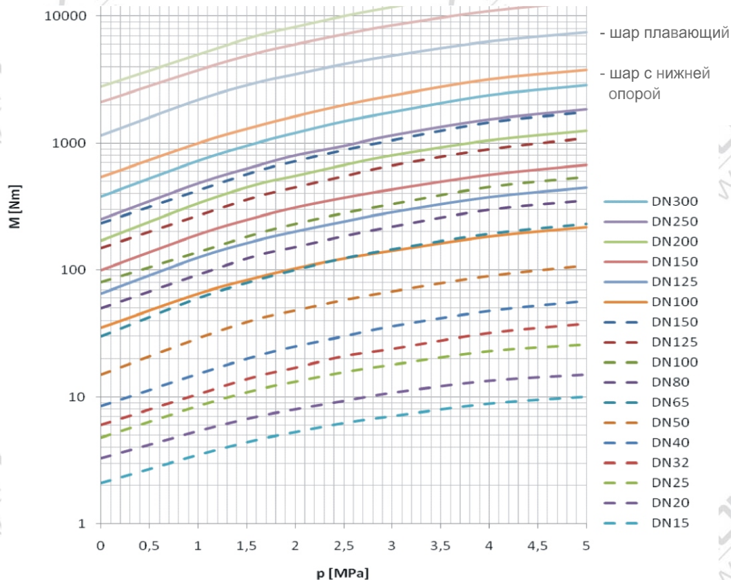
моменты открытия Opening torques
