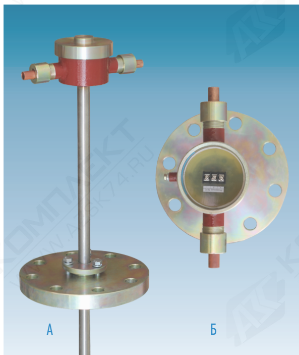
Рис. 1. Преобразователь магнитный поплавковый ПМП-118 (ПМП-138): А – внешний вид, Б – клеммный отсек.
