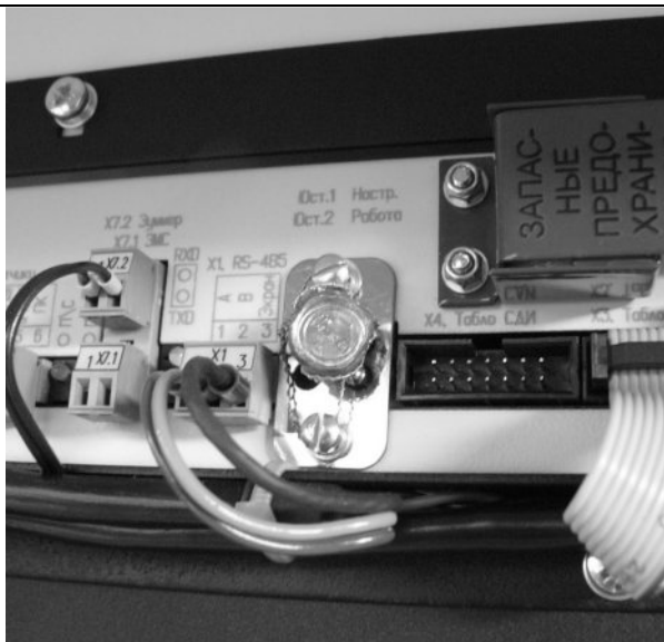
Рисунок В.2 Пломбировка блока управления
