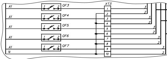
Схема подключения силовой части АЗС с ТРК "ТОПАЗ"
