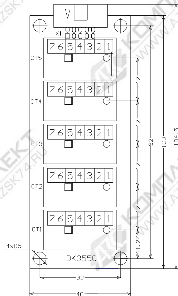
Рис. 43 Размеры модуля TOTM
