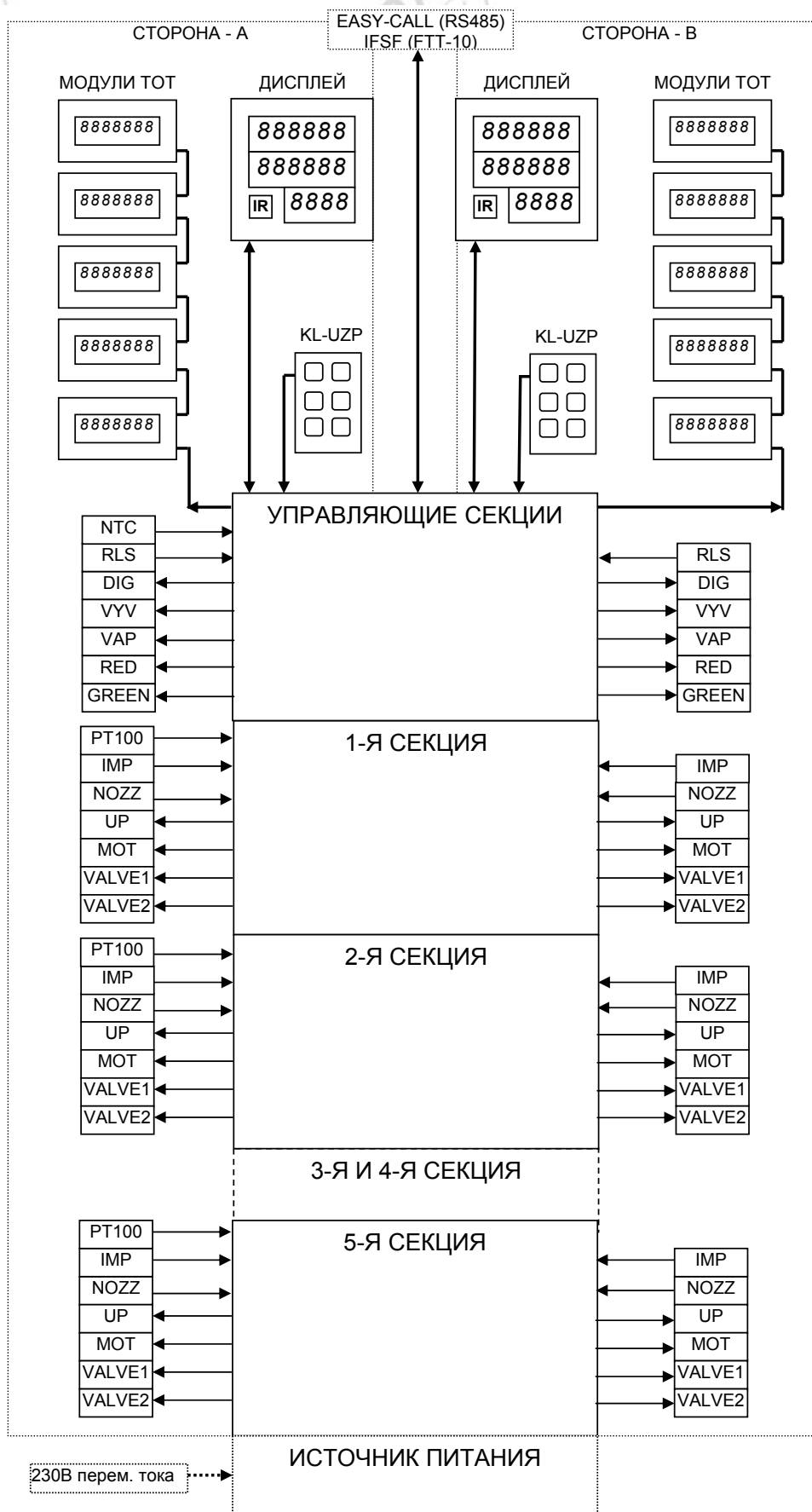
Рис. 1 Блок-схема счетчика ADPMPD/M
