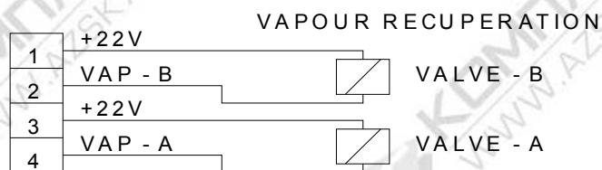
Рис. 36а Описание разъема X28
