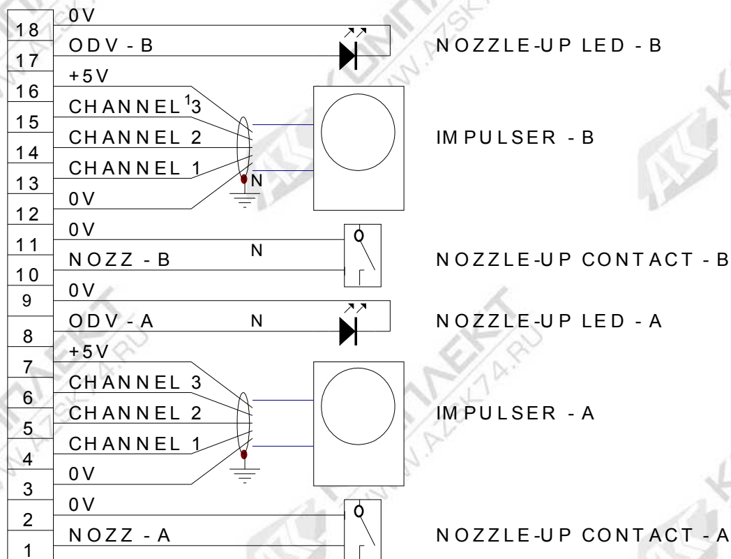
Рис. 31 Описание разъема X3
