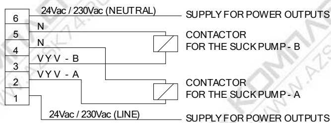
Рис. 32 Описание разъема X23
