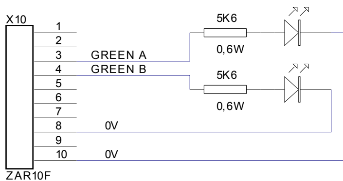
Рис. 36с Подключение LED для сигнализации большого расхода дизельного топлива
