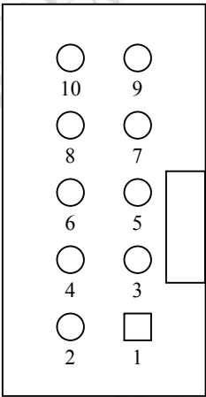
Рис. 30 Рисунок разъема X10
