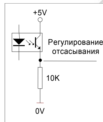
Рис. 3 Выход для регулирования отсасывания
