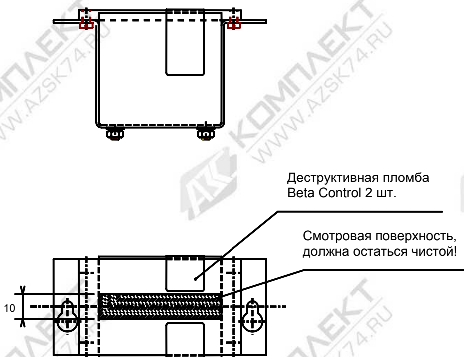
Рис. 42 Пломбирование модулей TOT
