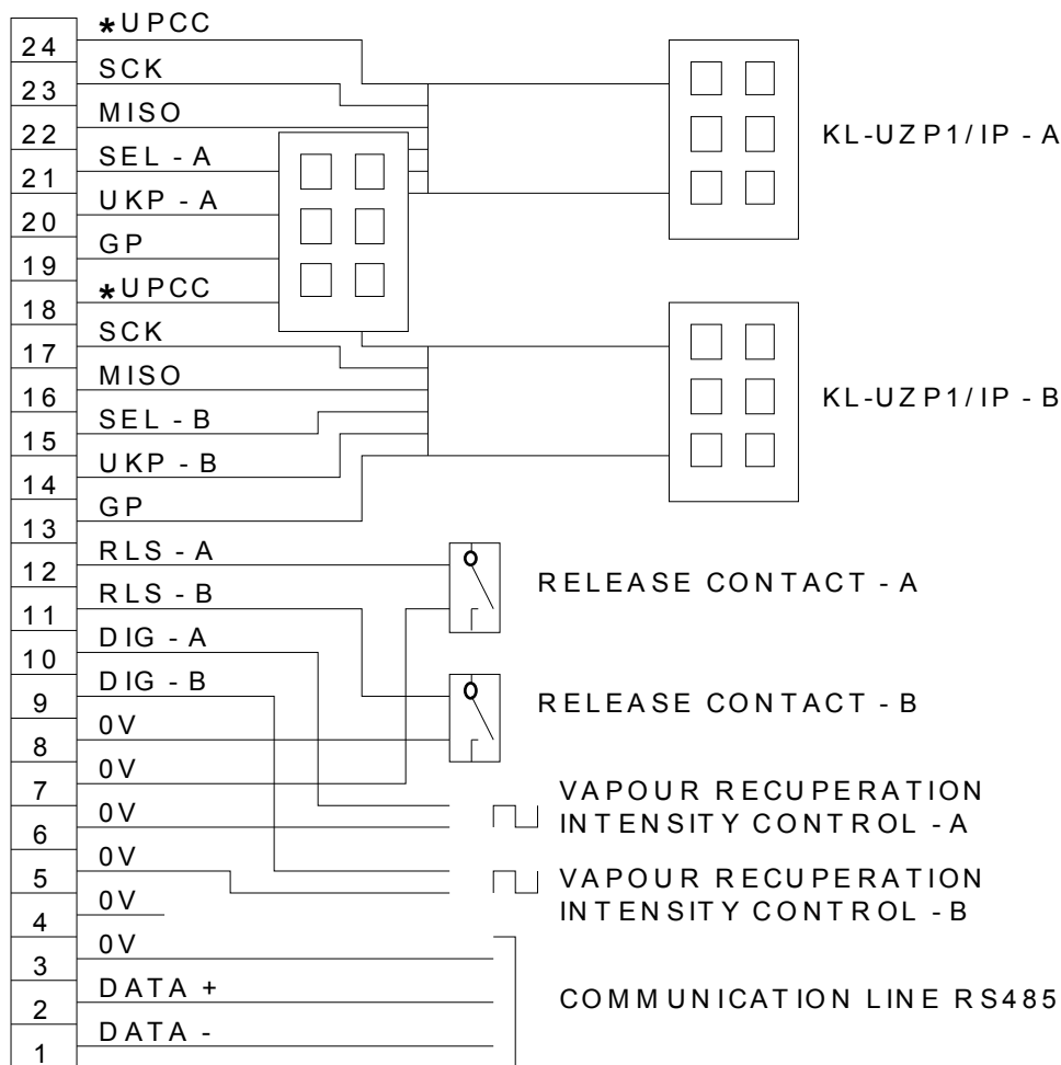
Рис. 34 Описание разъема X11
