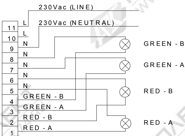
Рис. 35 Описание разъемов модуля SOPAM
