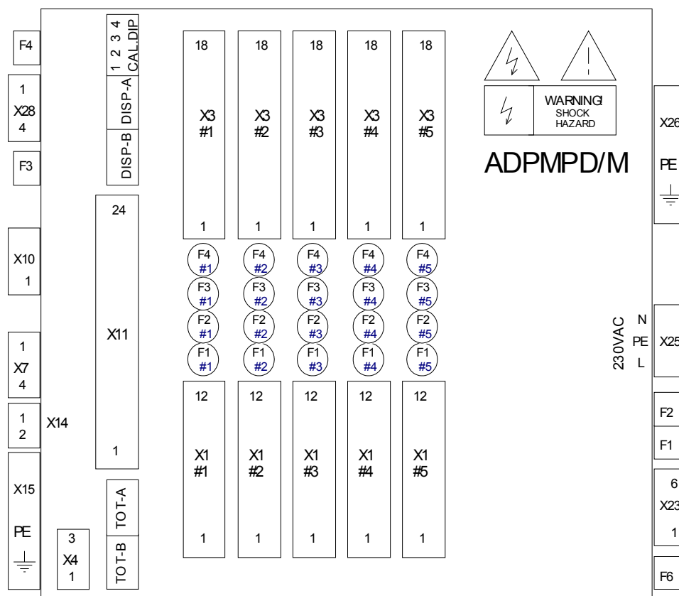
Рис. 28 Расположение разъемов ADPMPD/M
