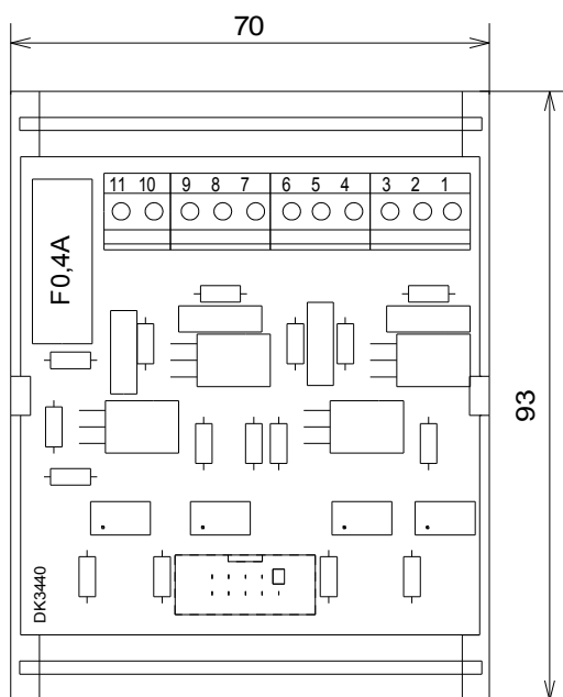
Рис. 44 Модуль SOPAM
