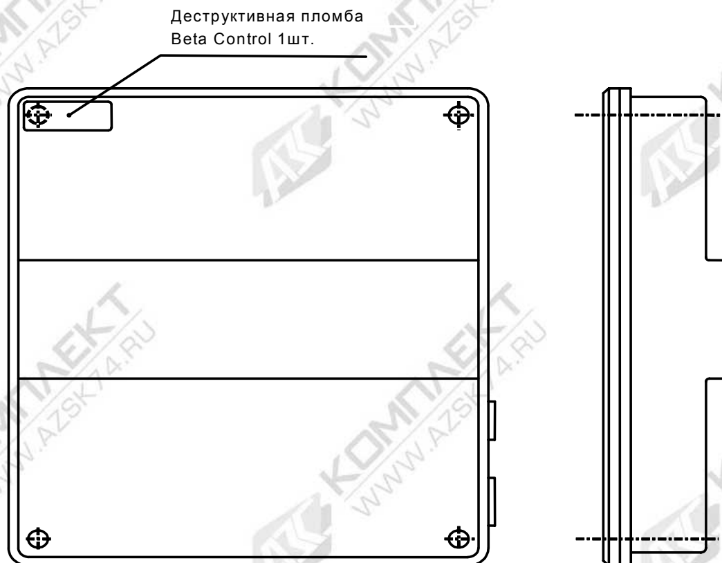
Рис. 41 Пломбирование дисплея на стороне колонки
