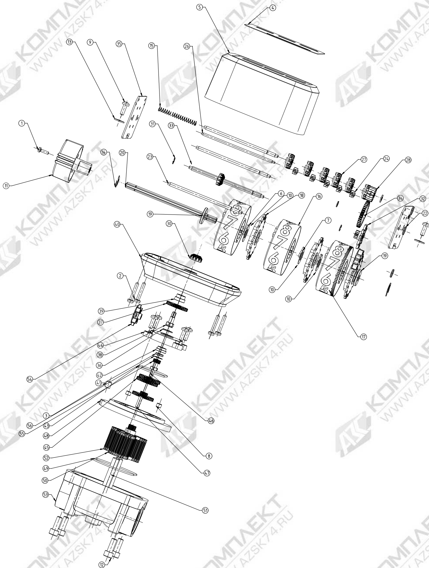
Рис 10-1: Схема составных частей счетчика на овальных колесах.
