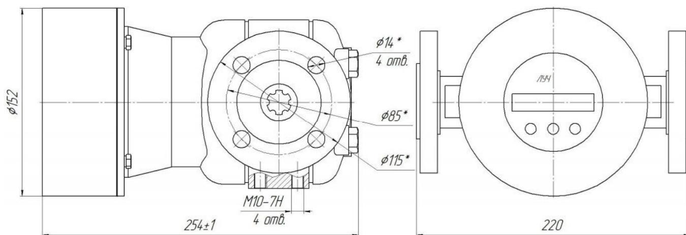
Рисунок Б.5 – Счётчик жидкости СЖ-ППО-25-1,6 ЛУЧ-03(штуцерный). Габаритные и присоединительные размеры
