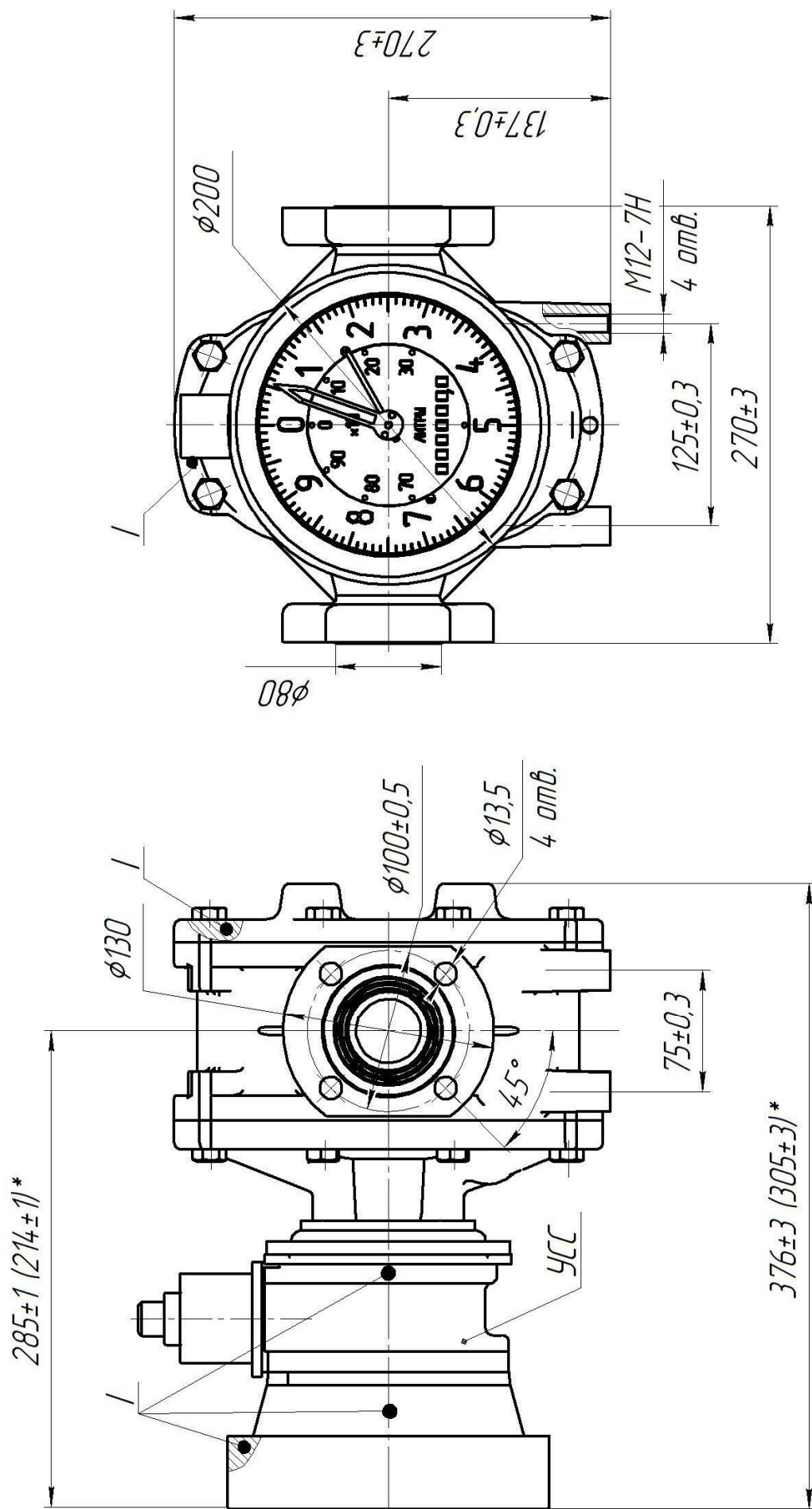
Рисунок Б.8 - Счётчик жидкости СЖ-ППО-40-0,6-УСС Б-25-СУ; Габаритные и присоединительные размеры
