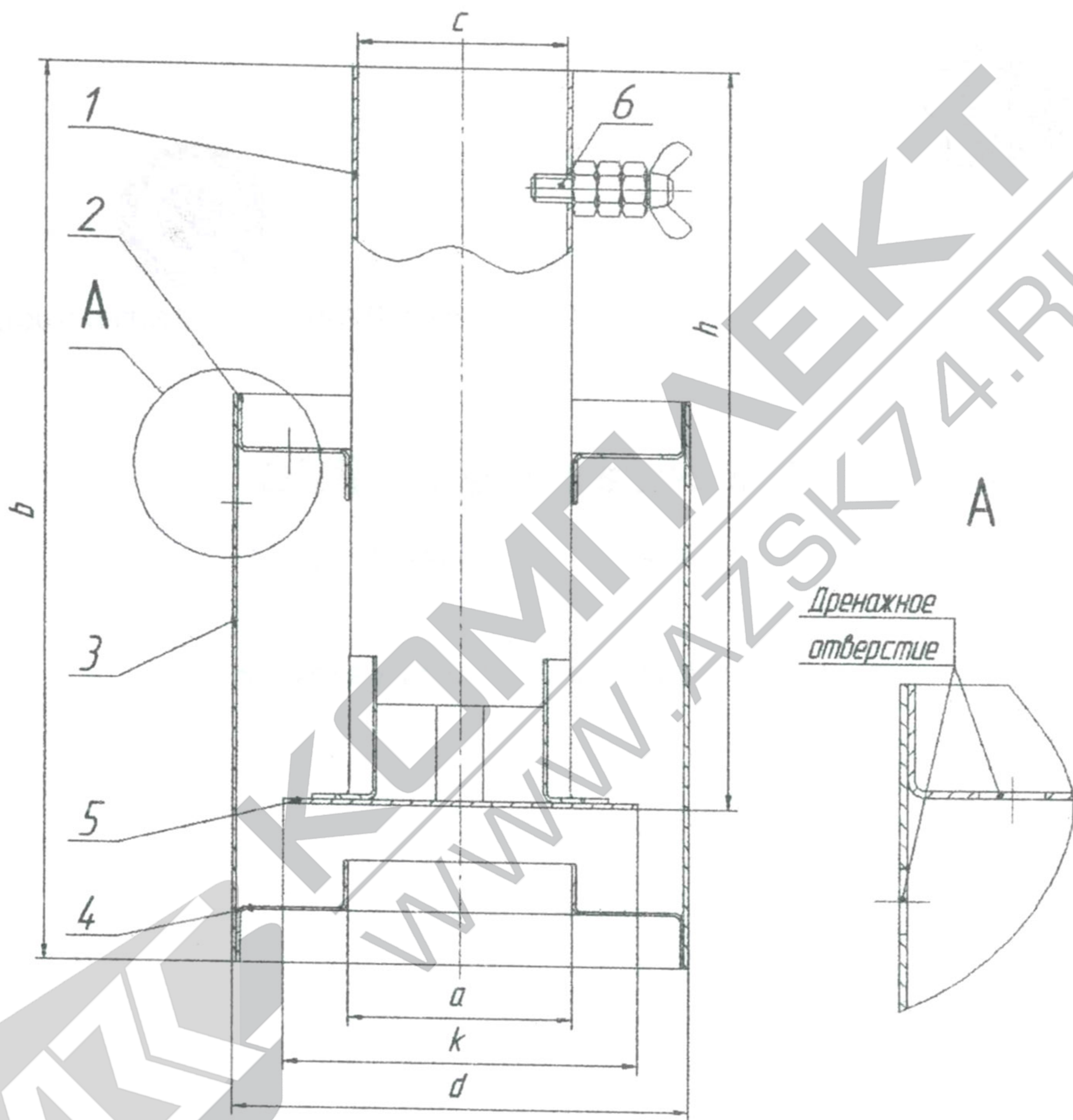
Рисунок 1. Общий вид.
