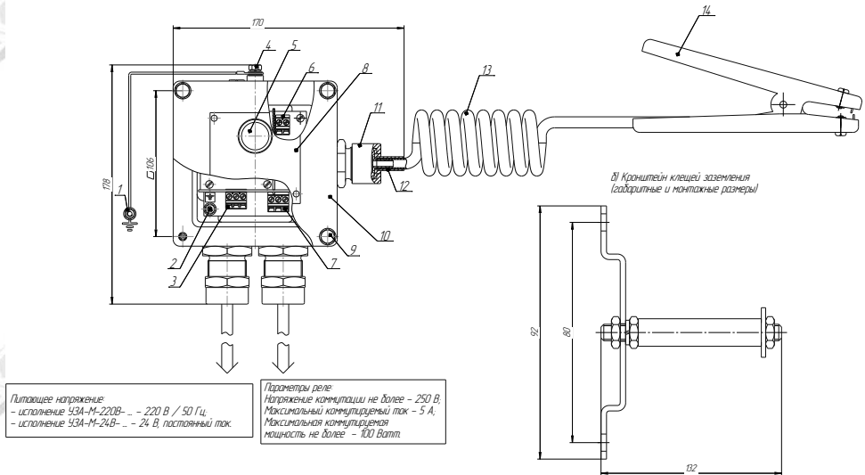
а) Устройство заземления автоцистерн УЗА-М...
