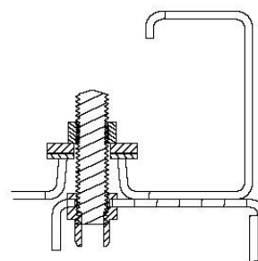
Сечение X-X
