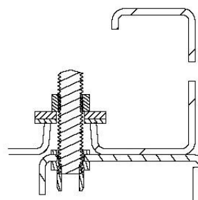
Сечение X-X
